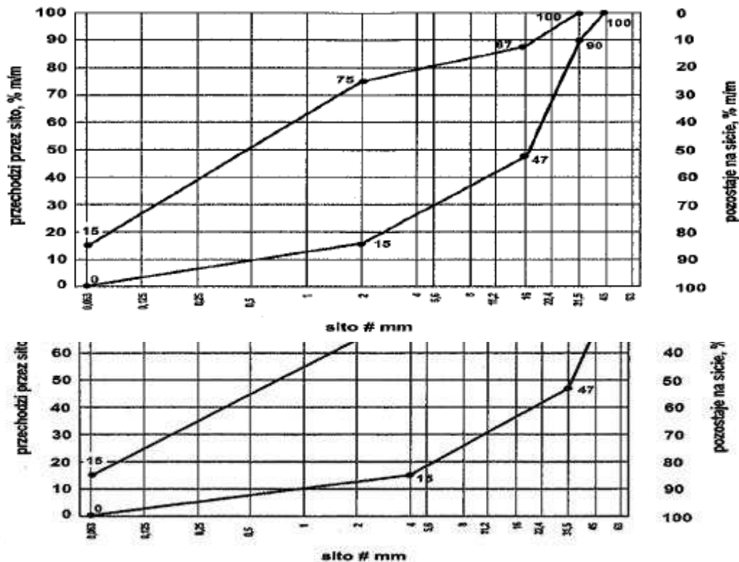
Rysunek 2. Mieszanka kruszywa 0/63 do górnej warstwy podłoża ulepszonych
