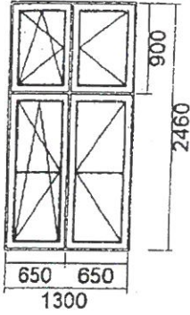
1) OKNO 2-SK.(słupek stały) (UR+R) 1300 x 2460
