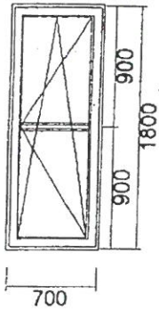
2) DRZWI BALK. 1-SK. (URP) 700 x 1800
